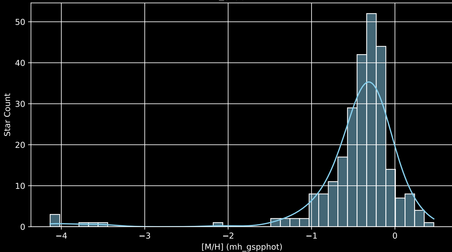
GALAH DR4 Field: [8896] [M/H] (mh_gspphot) (n= 260)
