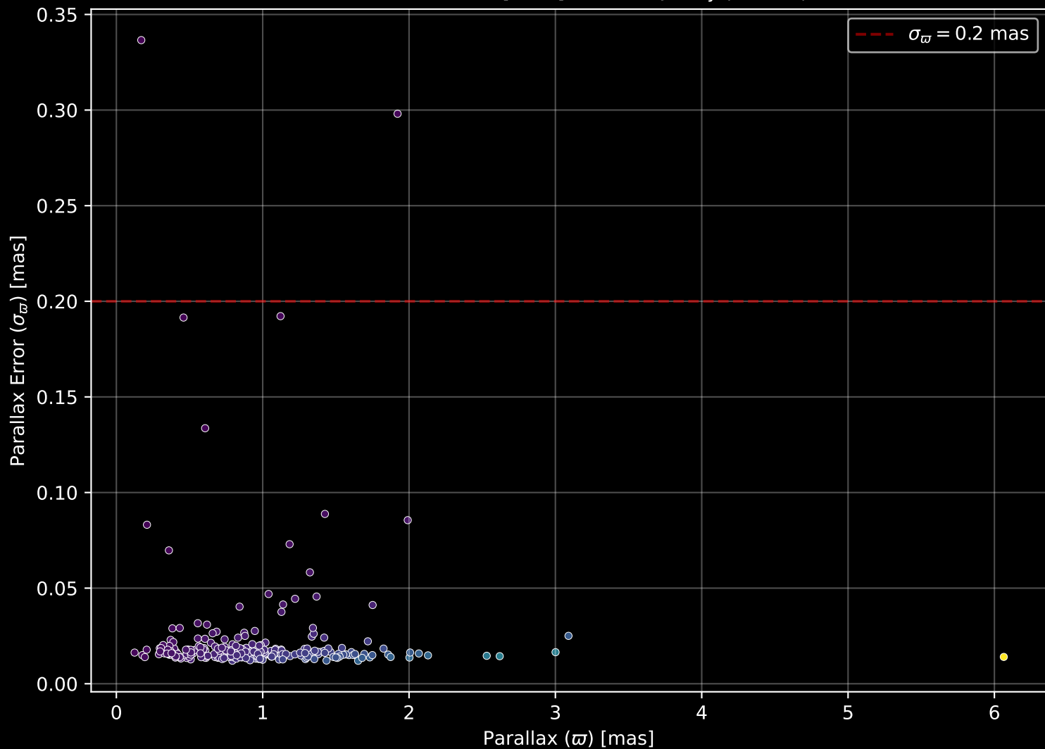
GALAH DR4 Field: [8896] Parallax Quality (n= 260)
