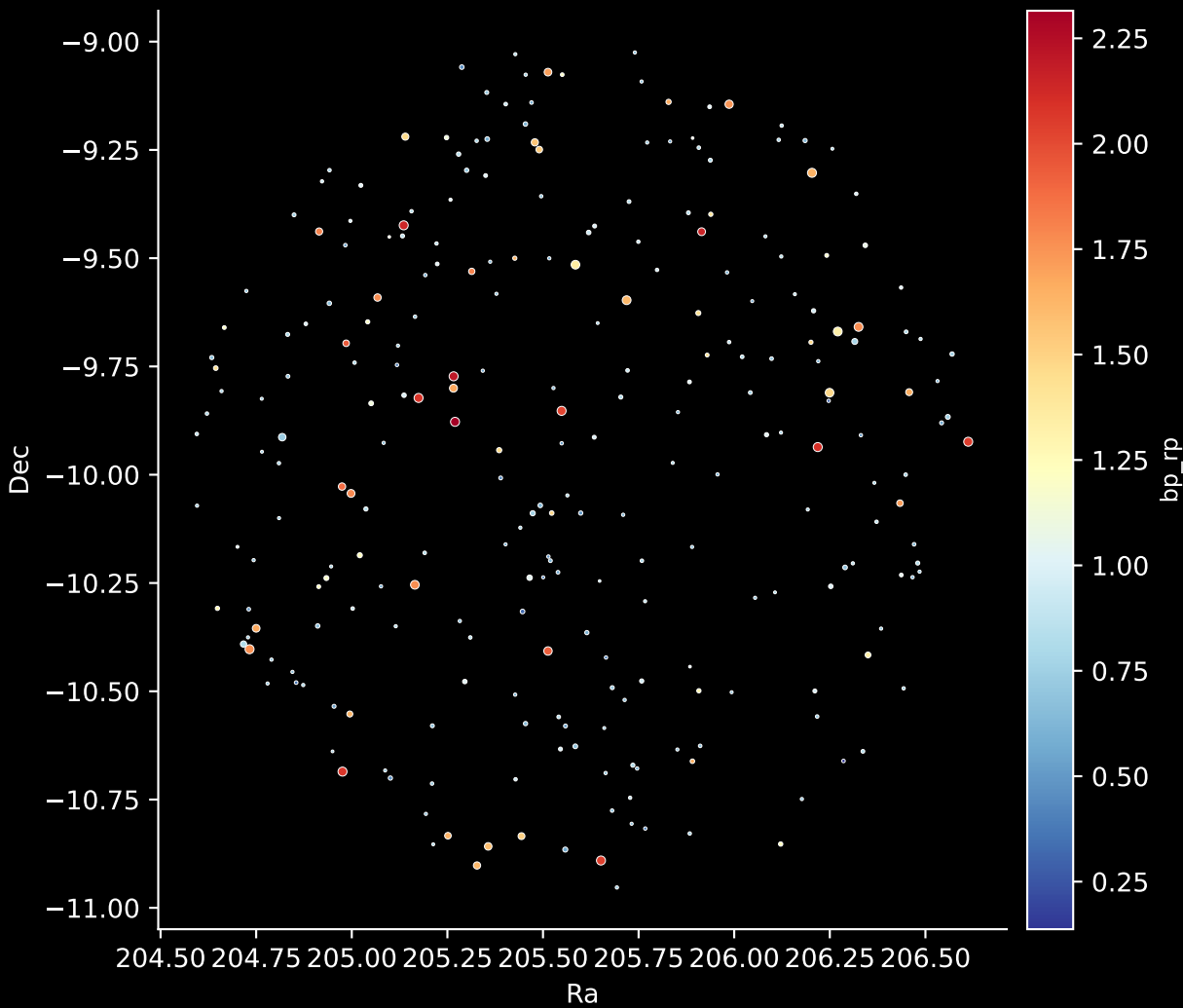
GALAH DR4 Field: [8896] Stars: 260
