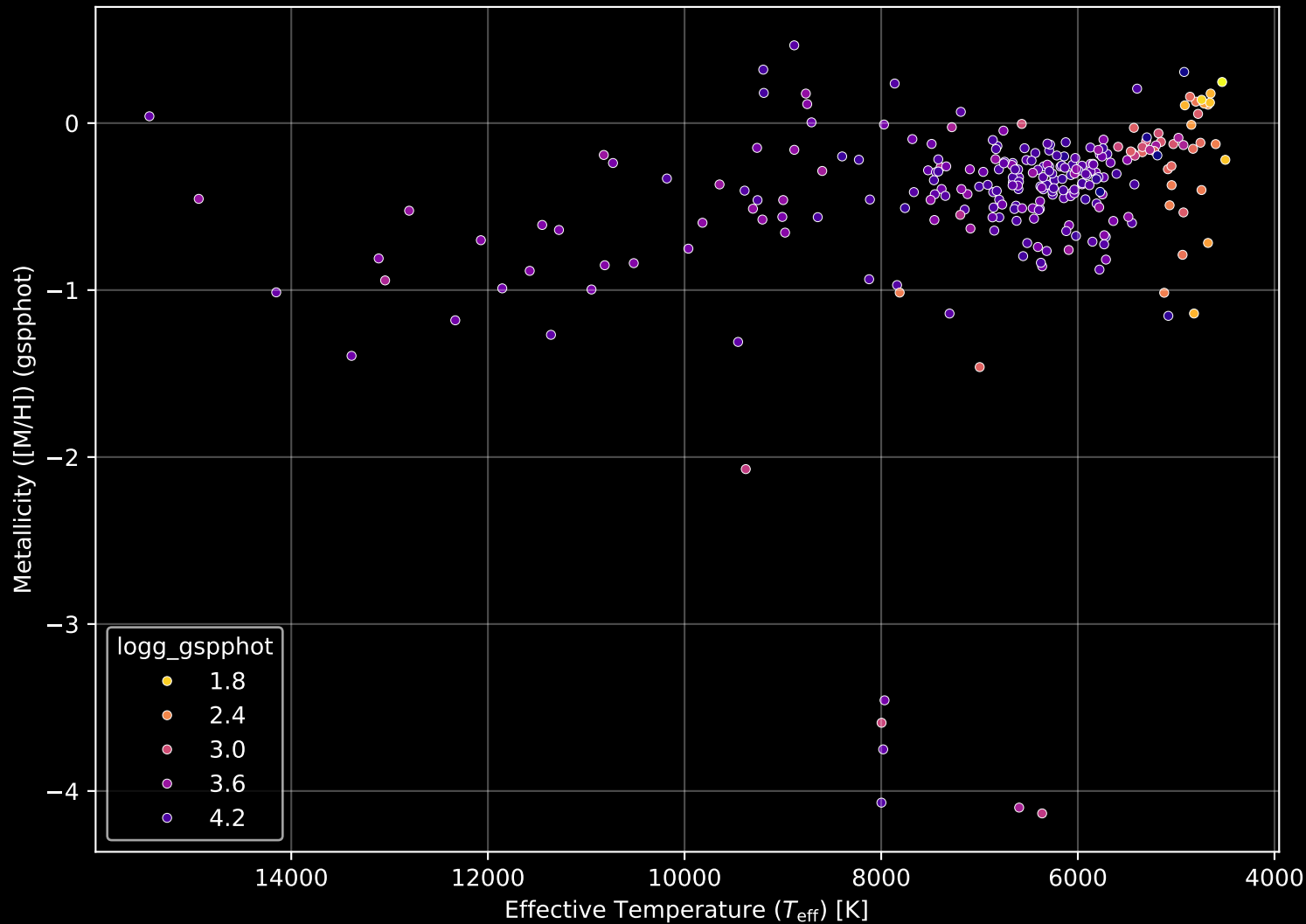
GALAH DR4 Field: [8896] Stellar Population Parameters (n= 260)
